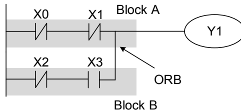
ORB(X0+X1), (X2+X3) Ladder diagram
