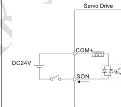
C10: Подключение входных сигналов (DI) с использованием внешнего источника питания
