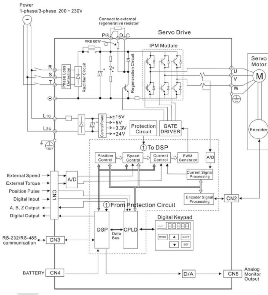
Рис. 3.5. Базовая схема соединений для моделей мощностью 750Вт (со встроенным тормозным резистором, но без вентилятора)
