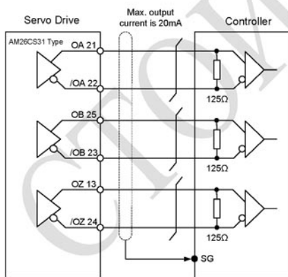
C13: Выходные сигналы энкодера (линейный драйвер)
