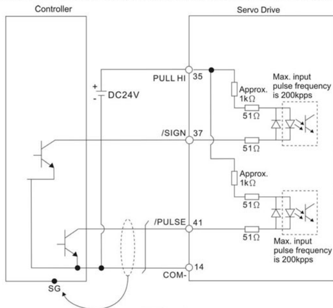
С3-2: Импульсы с открытого коллектора с использованием внешнего источника питания
