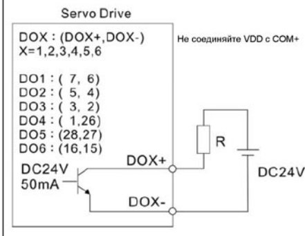
C7: Подключение выходных сигналов (DO) при использовании внешнего источника питания
