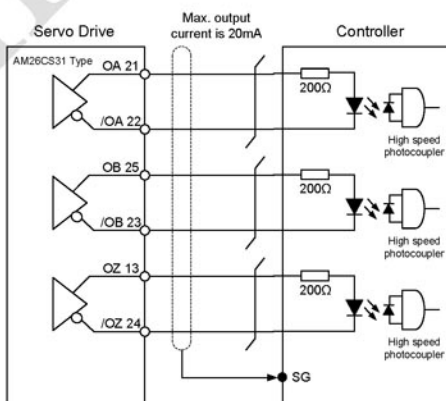
C14: Выходные сигналы энкодера (оптопара)
