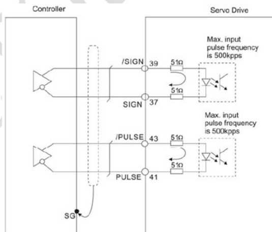
C4-1: Импульсный вход (Line driver). Требуется питание 5В. Запрещается подключать источник 24В.
