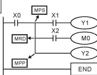
Релейно-контактная схема
