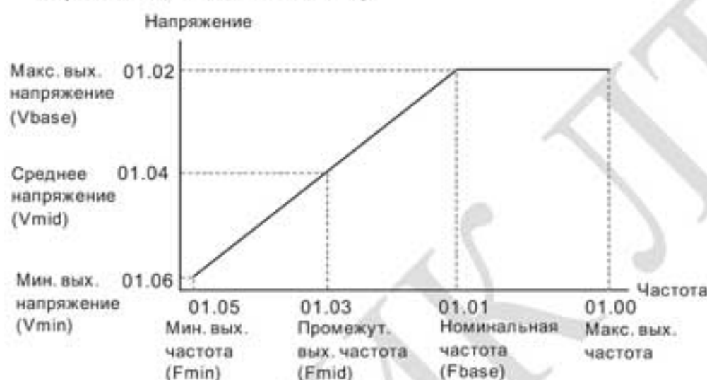
Кривая V/f
