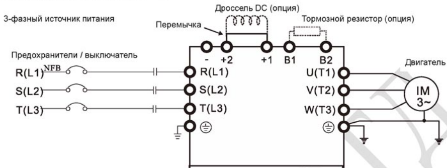
Рисунок 01: Типоразмеры A ~ C
