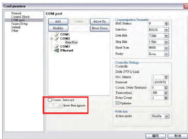
Рис. 3-4-3 Таблица коммуникационных настроек
