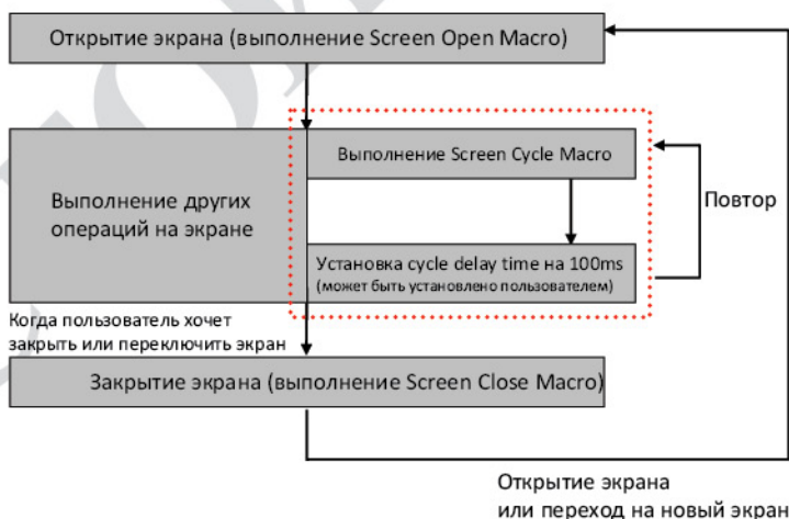
Рис. 3-14-2 Время задержки Macro Cycle
