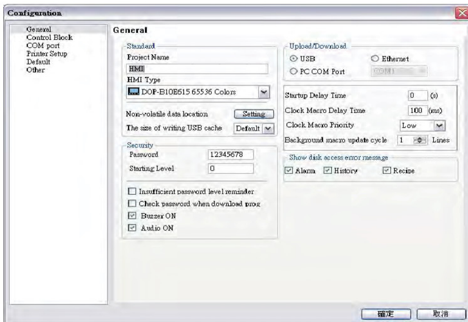
Рис. 3-5-11 Установка пароля –Security–
