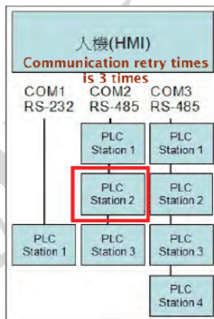
Рис. 3-4-4 Подключения ПЛК
