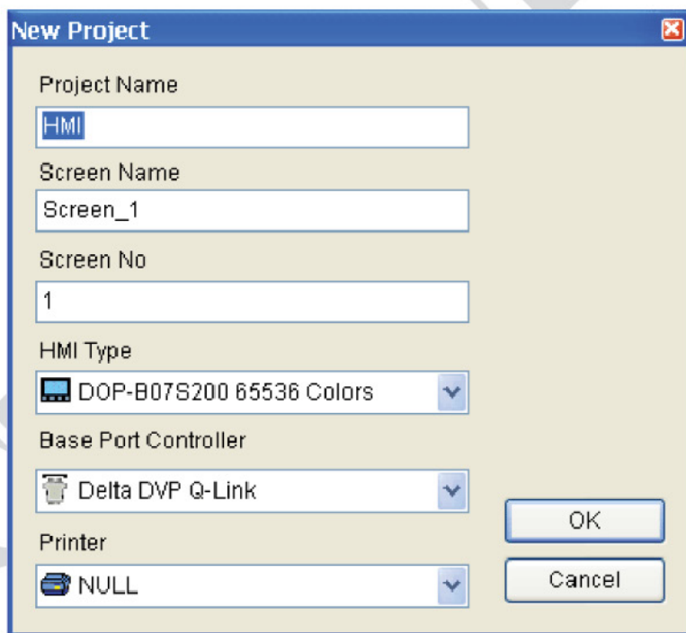
Рис.3.5.1 Новый проект. Открыть новый проект
