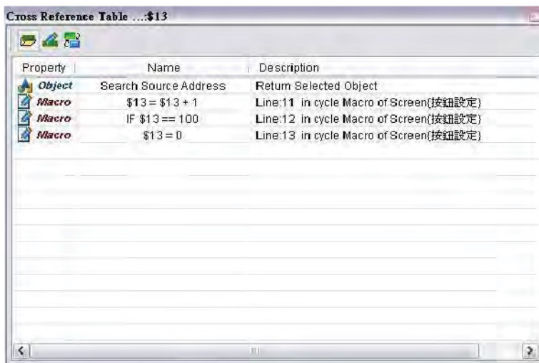
Рис. 3-7-15 Cross Reference Table
