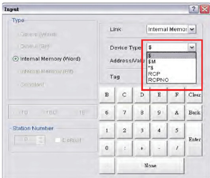
Рис. 3-3-1 Внутренняя память панели
