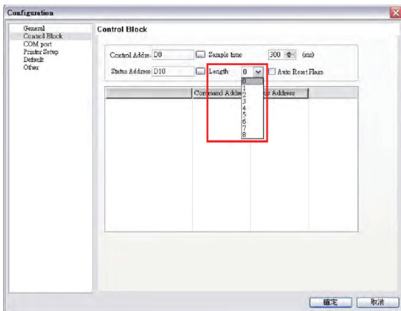
Рис. 3-4-2 Диалоговое окно Configuration
