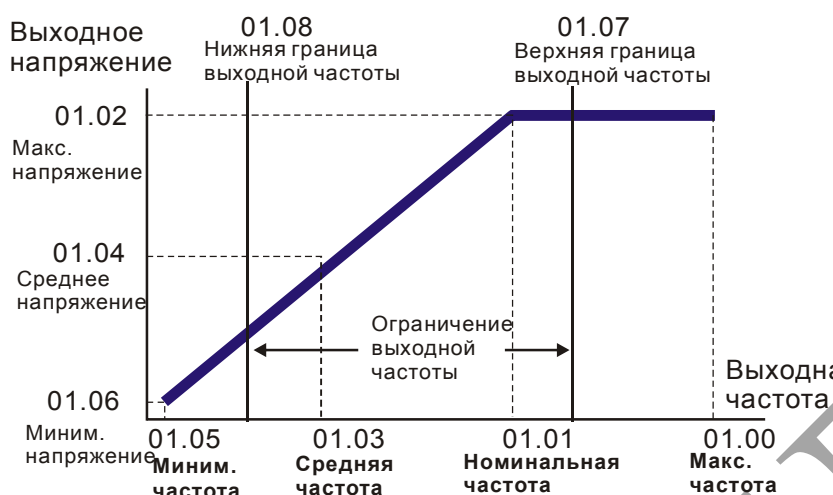
Типовая зависимость V/f
