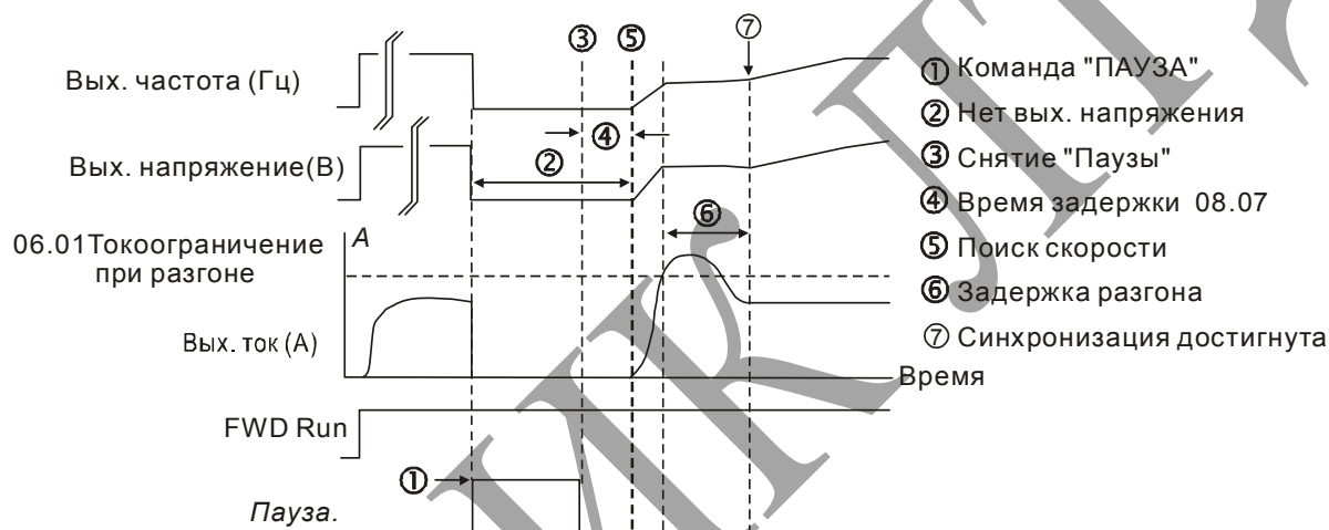
Рис 3: Поиск скорости с минимального значения частоты
