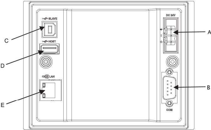
DOP-103BQ (Вид сзади)
