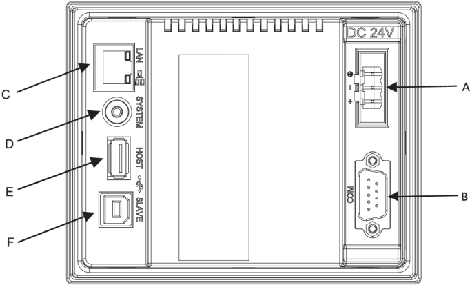
DOP-B03S(E)211 (Вид сзади)
